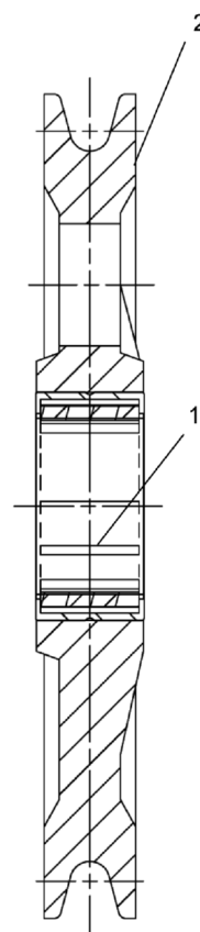
SECTION A-A
