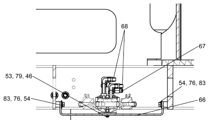
SECTION D-D
