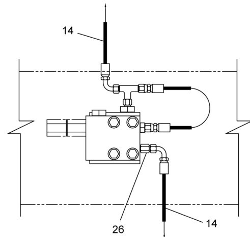
VIEW E - E
