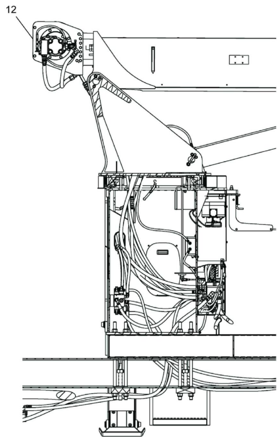
SECTION A-A
