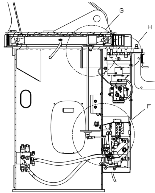
SECTION E - E
