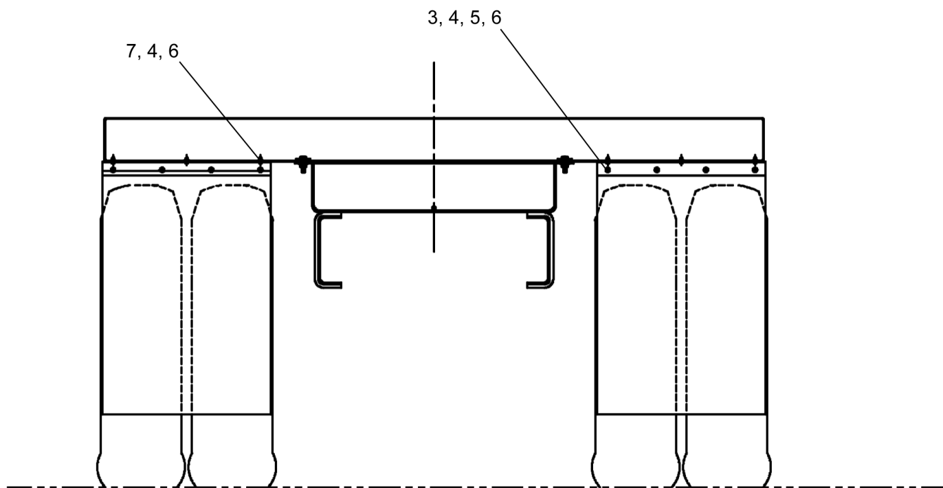
VIEW A-A
