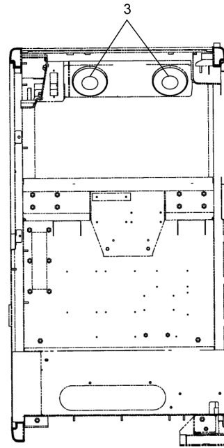
SECTION A-A
